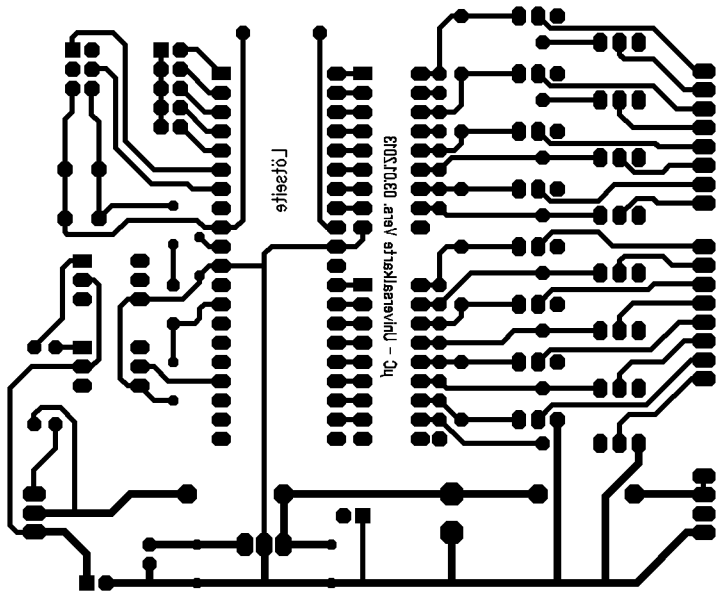
E516969 BOTTOM layer Image (topview)
