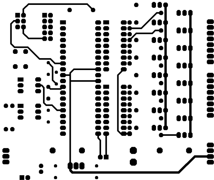
E516969 TOP layer Image (topview)
